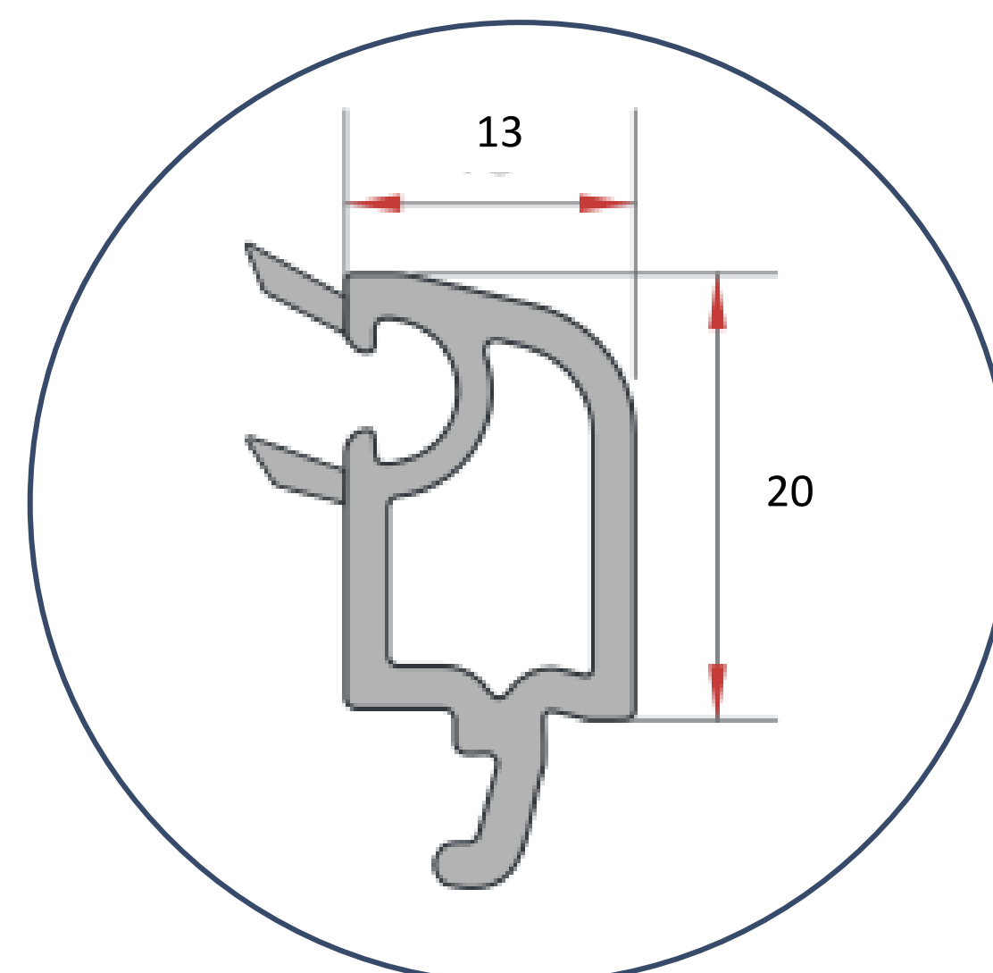
JUNQUILLO DOBLE CONTACTO TRIPLE ACRISTALAMIENTO 32 MM EN 48 0.225 GR/M
