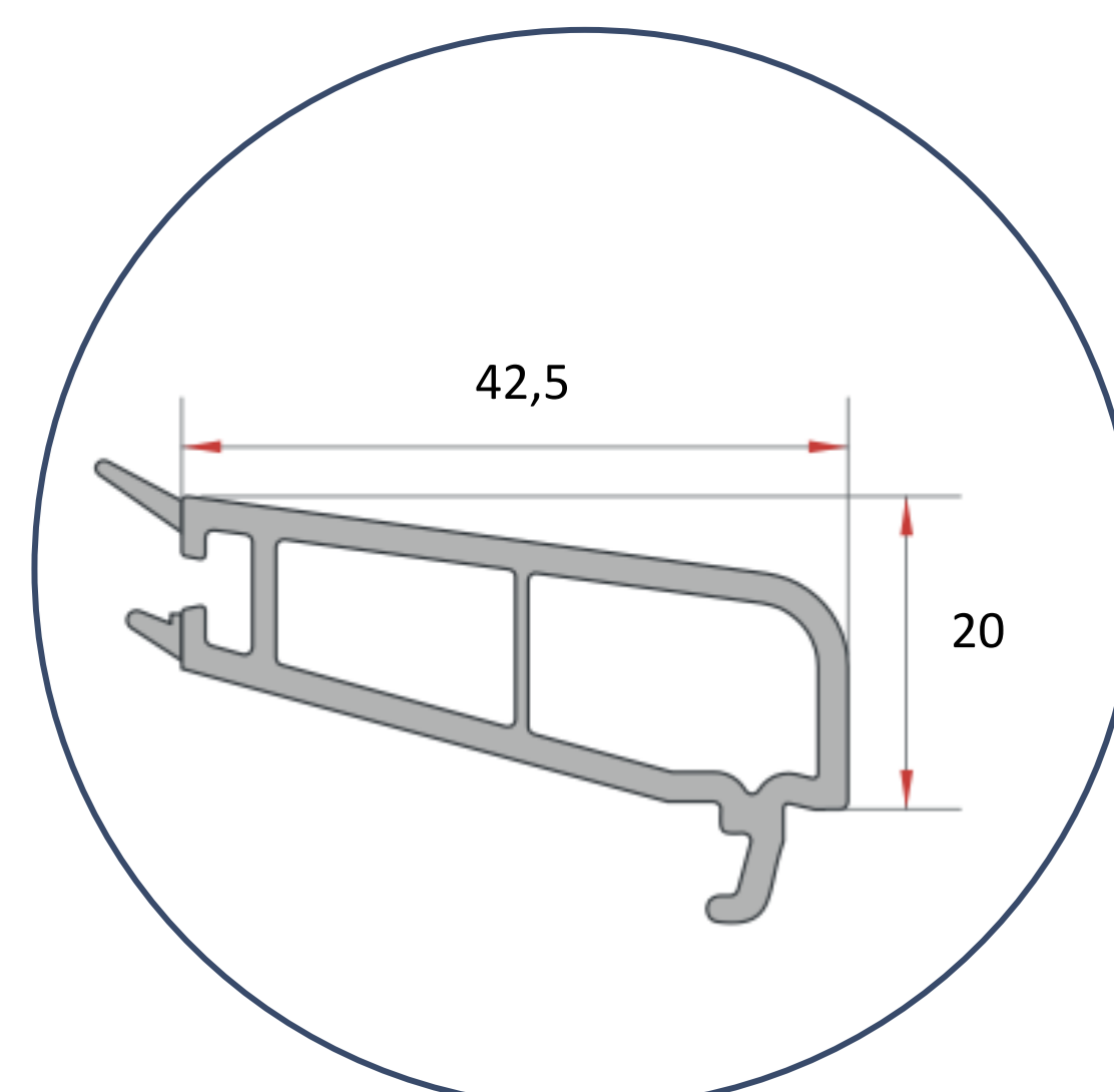
JUNQUILLO DOBLE CONTACTO ACRISTALAMIENTO 5 MM EN 45 0.250 GR/M
