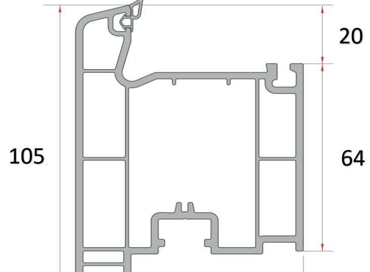
PERFIL HOJA PUERTA EN 21 1.465 GR/M
