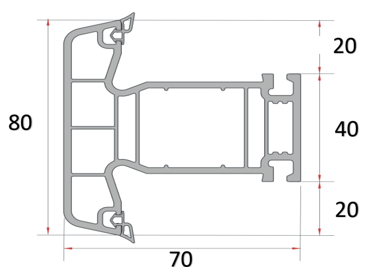
PERFIL PARTELUZ EN 17 1.335 GR/M
