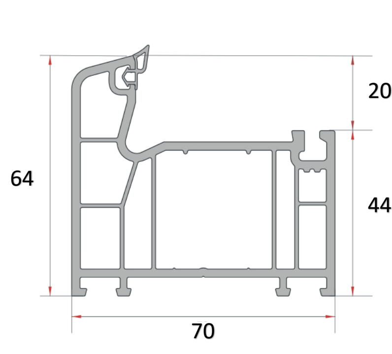
PERFIL DE MARCO EN 16 1.215 GR/M
