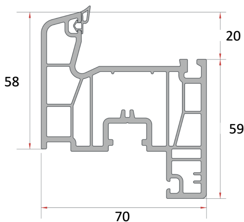
PERFIL HOJA PUERTA EXTERIOR EN 22 1.340 GR/M
