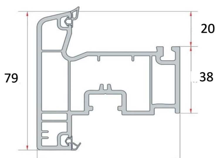
PERFIL MARCO EXTERIOR EN 23 1.340 GR/M
