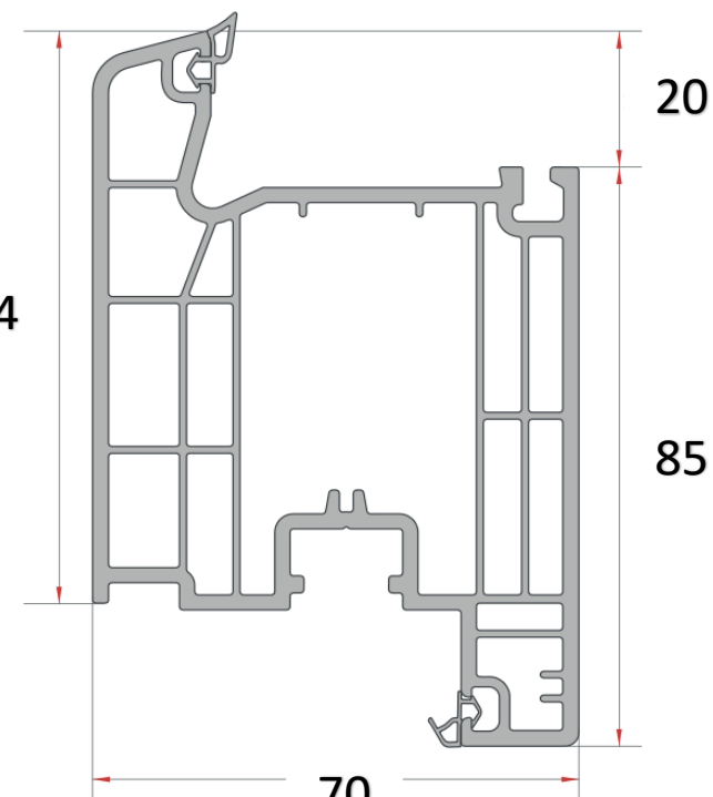
PERFIL HOJA PUERTA EN 21 1.830 GR/M
