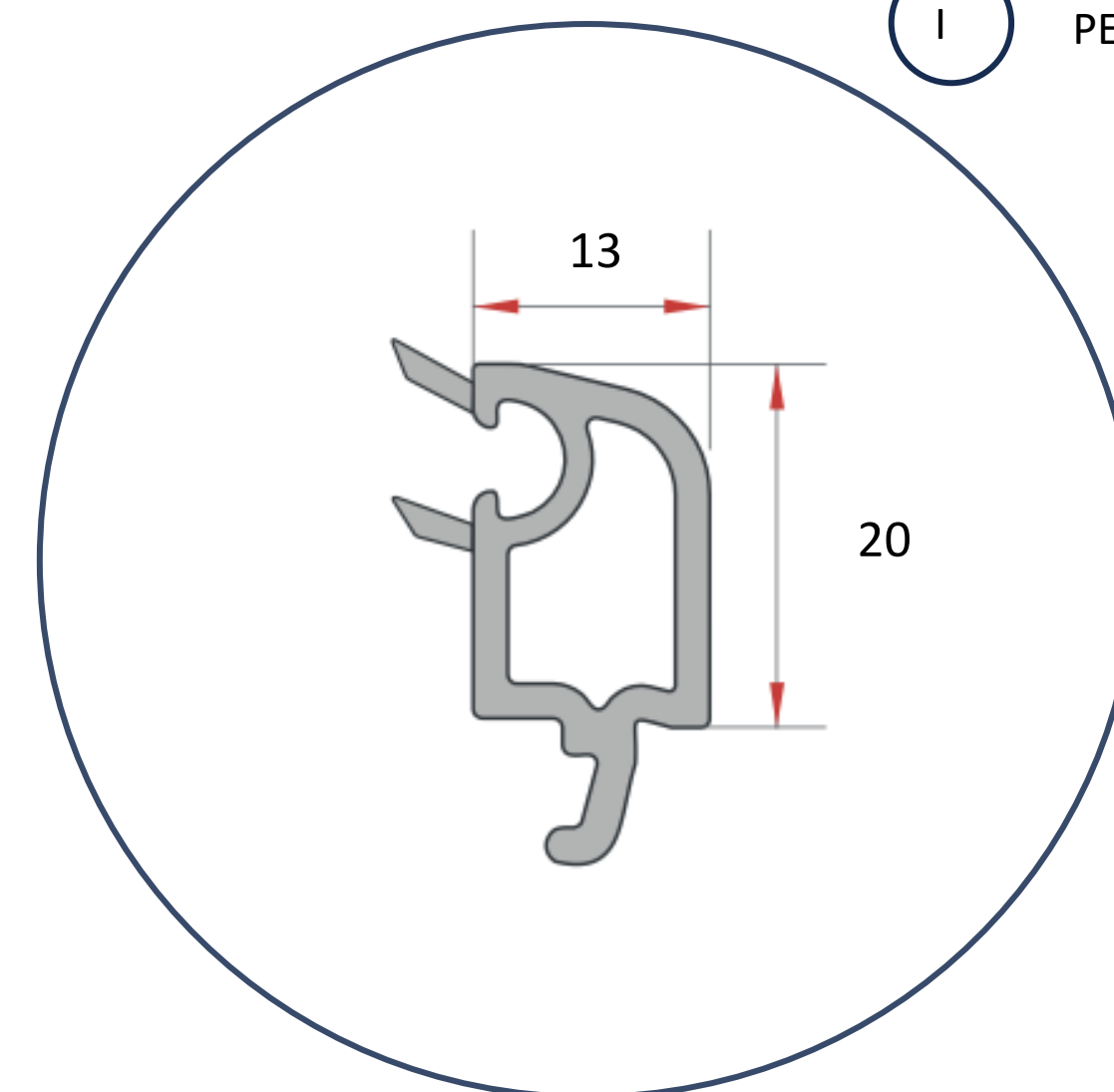
JUNQUILLO CORREDERA ACRISTALAMIENTO 20 MM EN 48 0.225 GR/M
