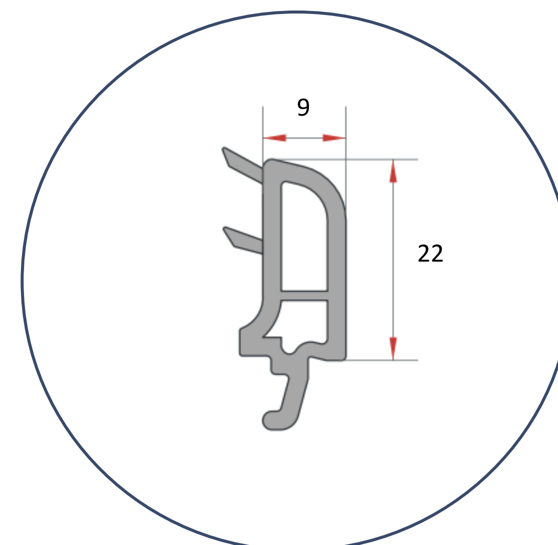
JUNQUILLO CORREDERA ACRISTALAMIENTO 24 MM EN 107 0.250 GR/M
