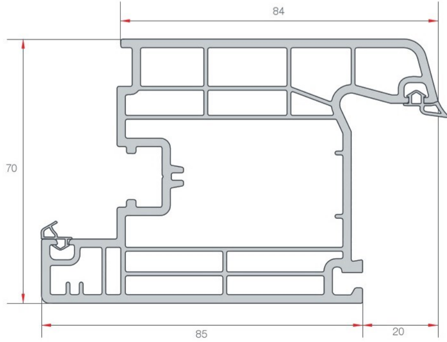
KAPI KANAT PROFİLİ DOOR SASH PROFILE EN 21 1.830 gr/m
