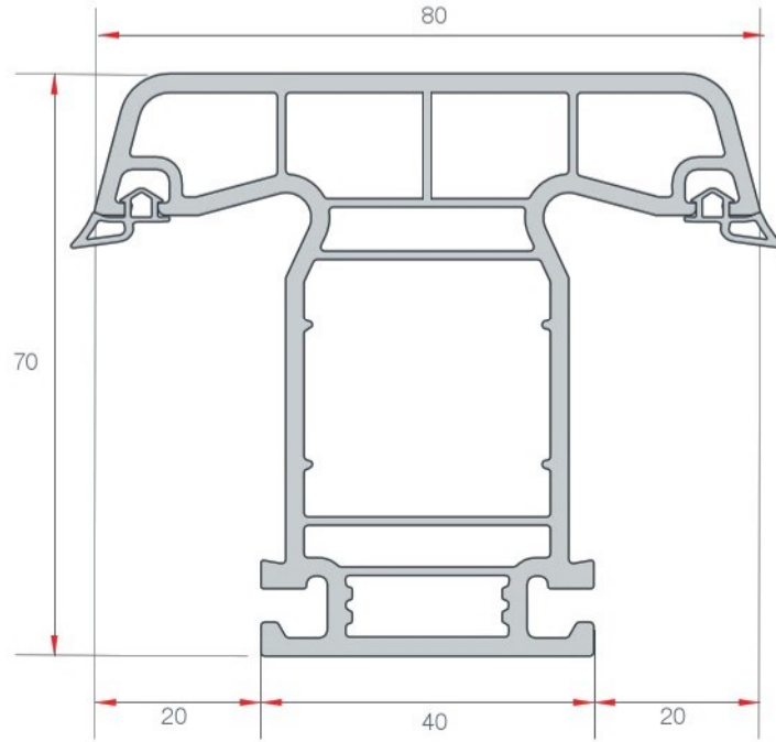
ORTA KAYIT PROFİLİ MULLION PROFILE EN 17 1.355 gr/m
