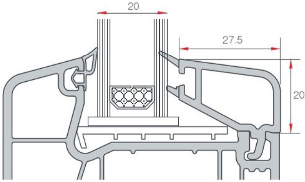
20 mm. ÇİFT CAM ÇİTASI DOUBLE GLAZING BEAD EN 45
