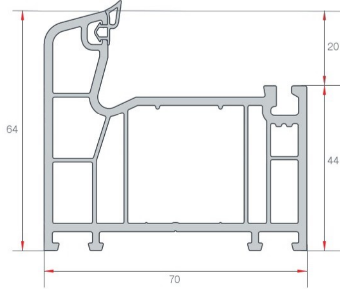
KASA PROFİLi FRAME PROFILE EN 16 1.215 gr/m
