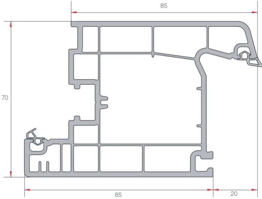
KAPI KANAT PROFİLİ DOOR SASH PROFILE EN 105 1.705 gr/m
